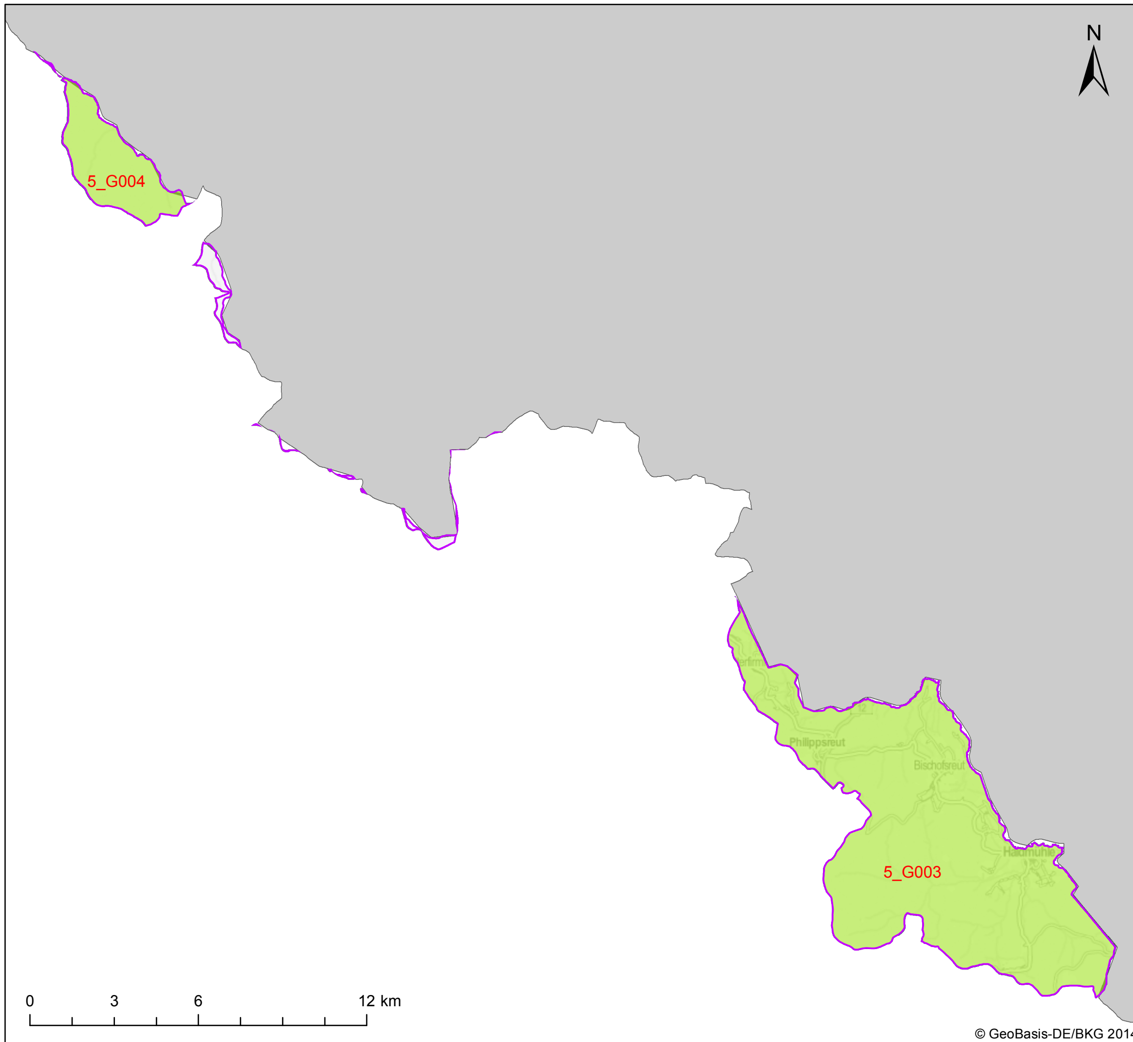
KOR Obere Moldau - Karte 4.6.1: Chemischer Zustand der Grundwasserkörper hinsichtlich Nitrat
