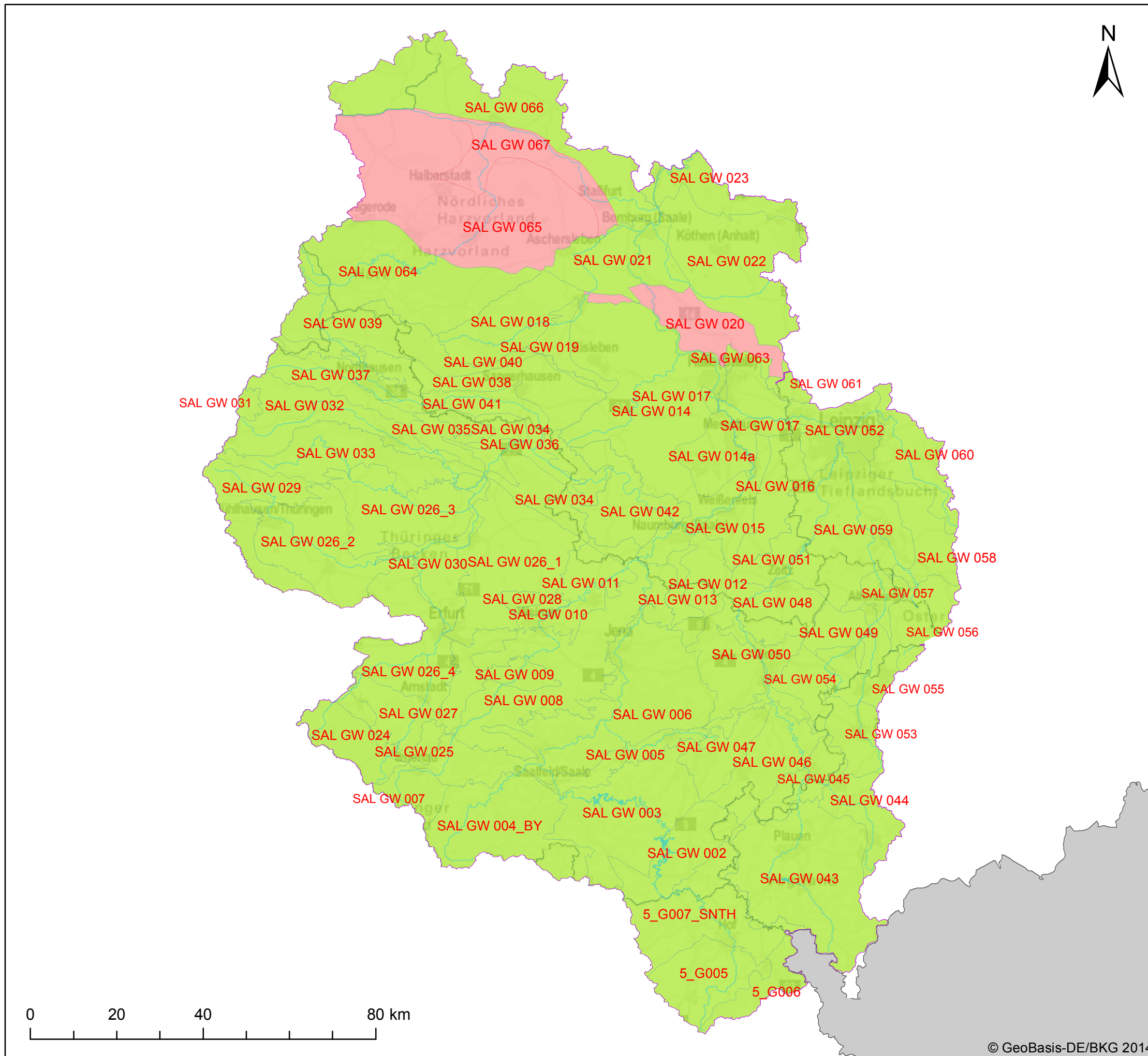
KOR Saale - Karte 4.6.2: Chemischer Zustand der Grundwasserkörper hinsichtlich Pestiziden
