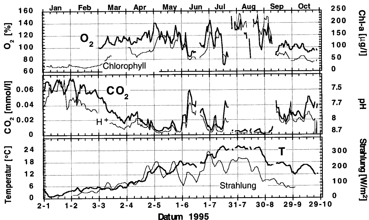
Abb. 12: Jahresgang (1995) der Tagesmittelwerte von O 2 -Sättigungsindex, Protonenkonzentrationen (pH-Wert), gelöstem CO 2 , Temperatur und Strahlung, Tagesmaximumwerte von Chlorophyll-a (Turner-Fluorimeter) am Wehr Geesthacht
