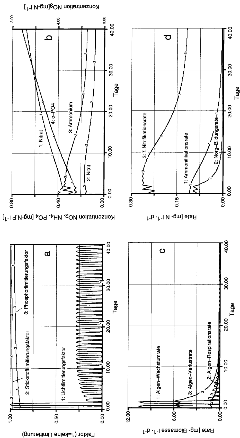
Abb. 31a-d: Modellierung eines Elbe-Längsprofils mit den Parametern von Abb. 29; Zu Abb. 30 gehörende Algen- und Stickstoffkomponenten
