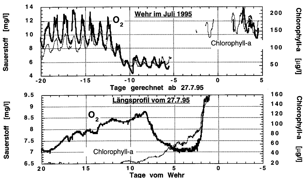
Abb. 24: Verlauf des Chlorophyll-a-Gehaltes und der \text{O}_2 -Konzentration vor dem 27. 7. 95 (27. 7. 95 = Zeitpunkt 0) am Wehr Geesthacht (A) und im Längsprofil (B). Das Längsprofil wurde mit mittleren Verweilzeiten für 400 \text{ m}^3/\text{s} von km in Zeit umgerechnet
