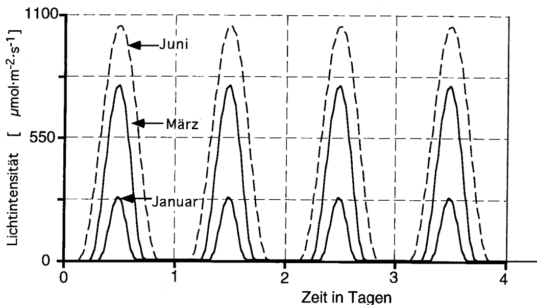
Abb. 27: Lichtfunktion für die Monate Januar, März und Juni
