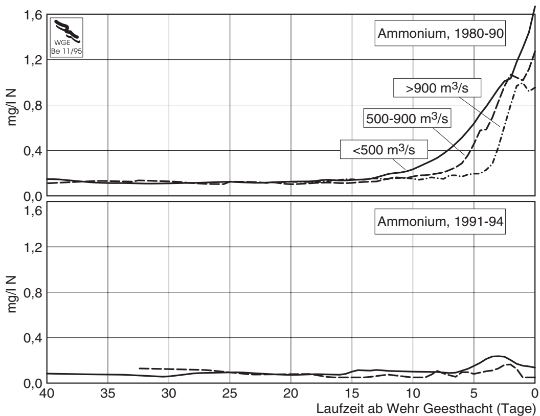
Abb. 22: Laufzeitnormierte, gemittelte Ammonium-Längsprofile der Elbe (Wassertemperatur T > 15^{\circ}\text{C} ) von 1980-1990 und von 1991-1994
