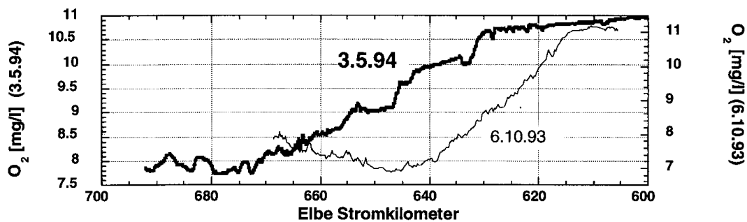
Abb. 18: O_2 -Gehalt im Längsprofil (km-Darstellung) bei unterschiedlichen Abflußbedingungen (Oberwasserabfluß am 6. 10. 93 = 365 m 3 /s, am 3. 5. 94 = 1350 m 3 /s)
