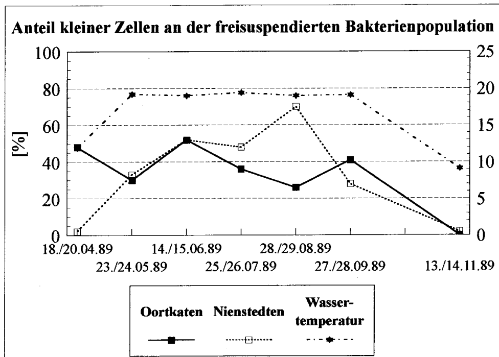
Abb. 7: Prozentualer Anteil von kleinen Zellen (Durchmesser: < 0,4 \mu\text{m} ) an der freisuspendierten Bakterienpopulation von Wasserproben der Stationen Oortkaten und Nienstedten von Mai 1989 bis November 1989
