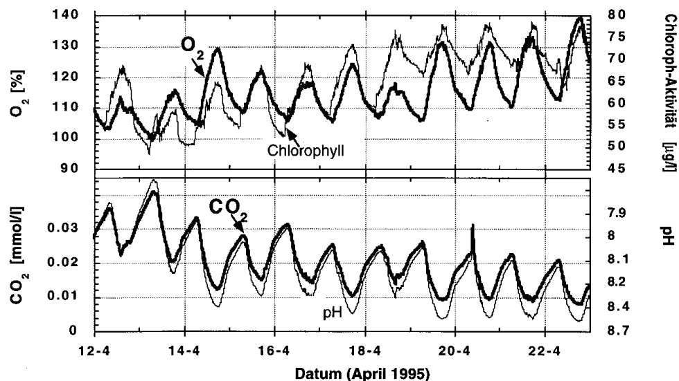
Abb. 11: Tagesgänge von \text{O}_2 -Sättigungsindex, Chlorophyll-a-Aktivität (Turner-Fluorimeter), Protonenkonzentrationen (pH-Wert) und gelöstem \text{CO}_2 am Wehr Geesthacht im April 1995
