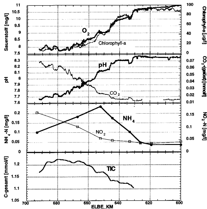
Abb. 16: Kontinuierliche Messung von Chlorophyll-a (Turner), O 2 , CO 2 und pH-Wert, Ammonium und Nitrit aus Einzelproben, TIC (total inorganic carbon) (aus pH und CO 2 berechnet) – Elbelängsprofil vom 3. 5. 94 (Abfluß 1350 m 3 /s)
