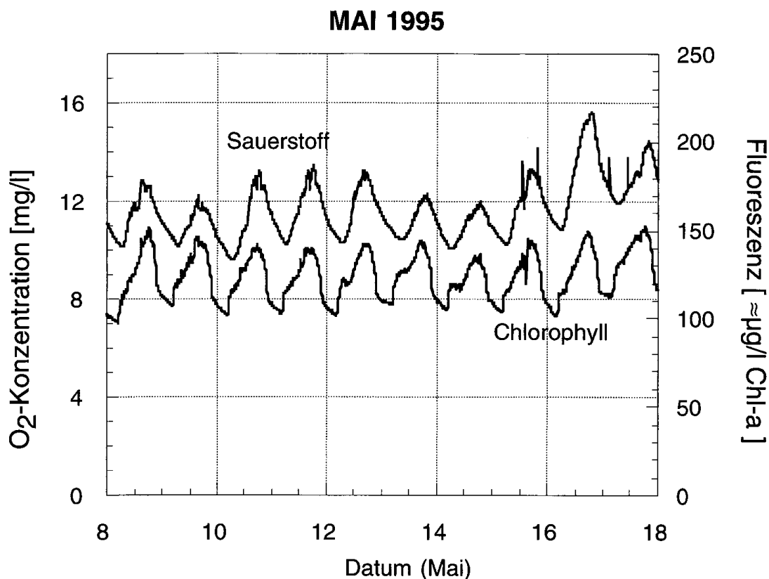
Abb. 28: Kontinuierlich gemessene Sauerstoff- und Chlorophyllkonzentrationen am Wehr Geesthacht im Mai 1995 (Chlorophyll über die prompte Fluoreszenz)
