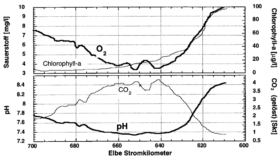
Abb. 15: Kontinuierliche Messung von Chlorophyll-a (Turner), O_2 , CO_2 und pH-Wert – Elbe-Längsprofil vom 5. 8. 93 (Abfluß 500 \text{ m}^3/\text{s} )
