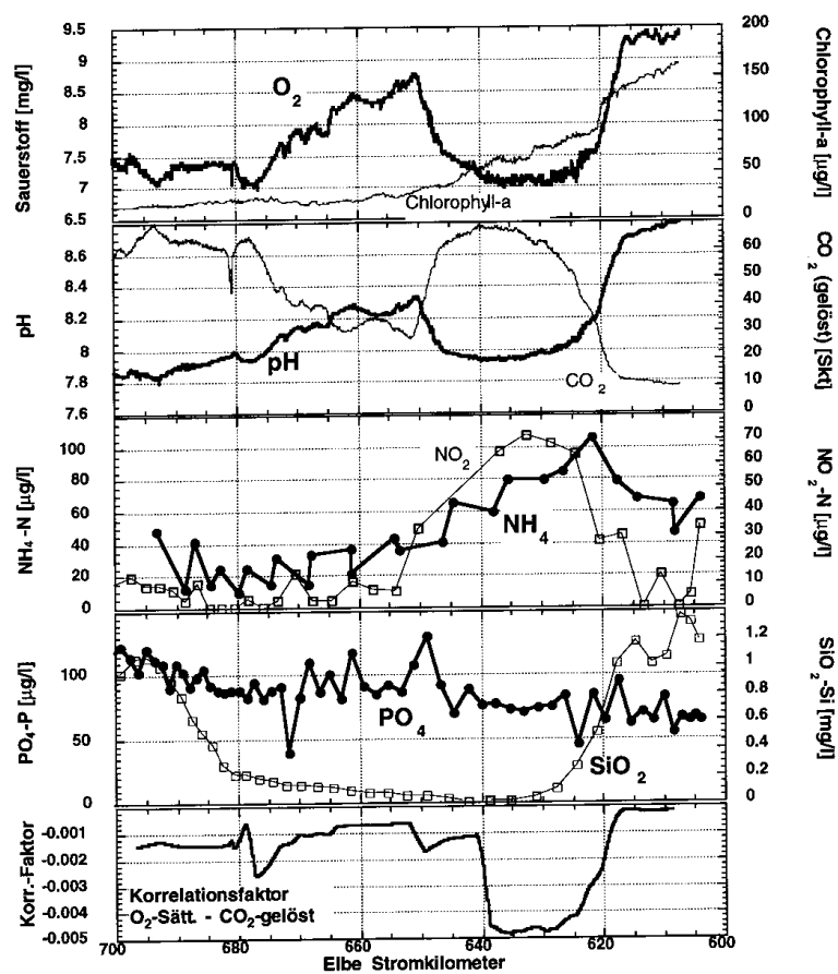
Abb. 23: Kontinuierlich gemessene Konzentrationen (Chlorophyll-a (Turner), \text{O}_2 , \text{CO}_2 , pH, Ammonium, Nitrit, Phosphat, Silikat) im Elbelängsprofil am 27. 7. 95 sowie funktioneller Zusammenhang (Korrelationsfaktor) zwischen \text{O}_2 -Sättigungsindex und gelöstem \text{CO}_2 (Korrelationsfaktor abschnittsweise berechnet)
