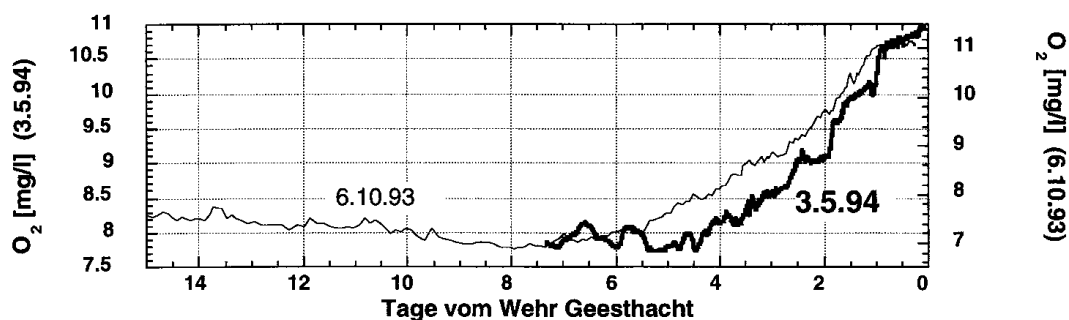
Abb. 19: O_2 -Gehalt im Längsprofil (Zeit-Darstellung) bei unterschiedlichen Abflußbedingungen (Oberwasserabfluß am 6. 10. 93 = 365 m 3 /s, am 3. 5. 94 = 1350 m 3 /s)
