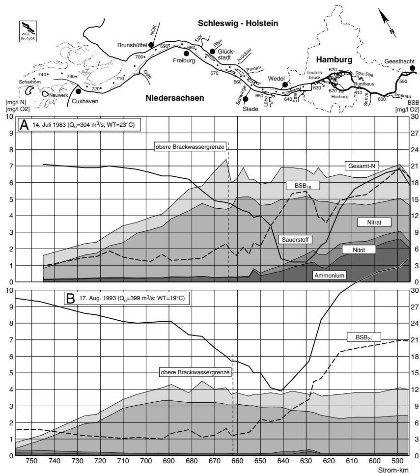
Abb. 9: Ammonium-, Nitrit-, Nitrat- (gestapelt) und Gesamt-Stickstoff-, BSB 15 bzw. BSB 21 - und Sauerstoffgehalte im Längsprofil der Tideelbe. A: 14. Juli 1983, B: 17. August 1993
