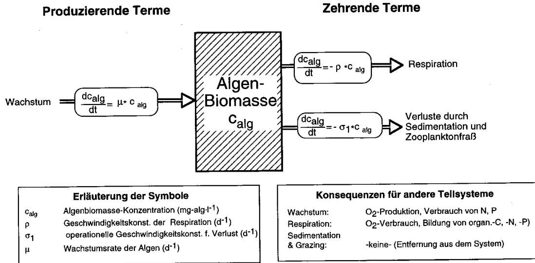
Abb. 25b: Im Modell berücksichtigte Prozesse des Teilsystems „Algenbiomasse“
