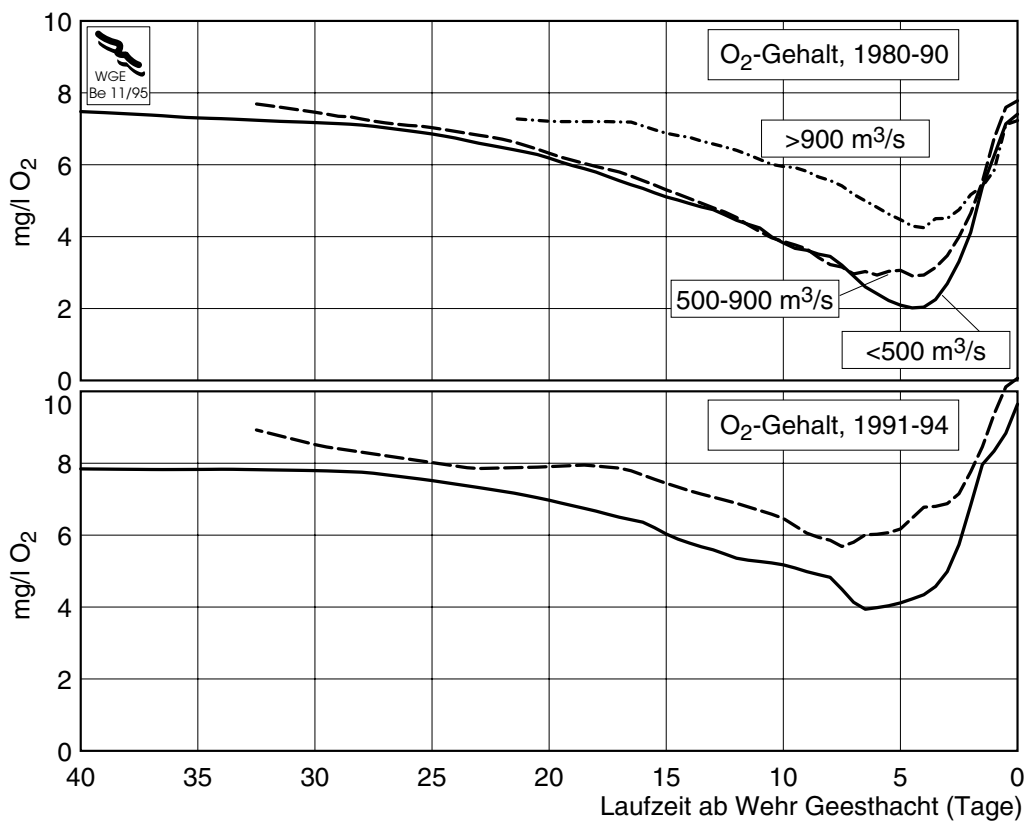
Abb. 20: Laufzeitnormierte, gemittelte O_2 -Längsprofile der Elbe (Wassertemperatur T > 15^\circ C ) von 1980-1990 und von 1991-1994
