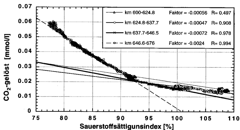
Abb. 17: Korrelation \text{CO}_2 -Sauerstoffsättigungsindex für verschiedene km-Abschnitte im Elbe-Längsprofil vom 3. 5. 94
