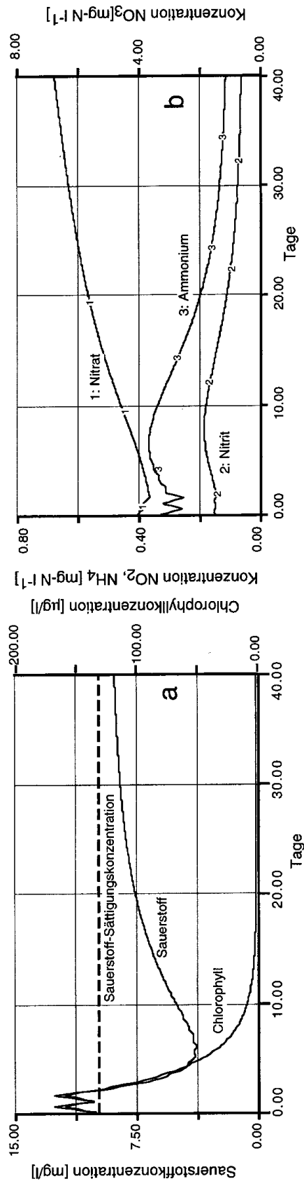
Abb. 32: Modellauf mit den Parametern wie in Abb. 29, jedoch Änderung des Verhältnisses Algenverluste : Algenrespiration (s. Tab. 4)
