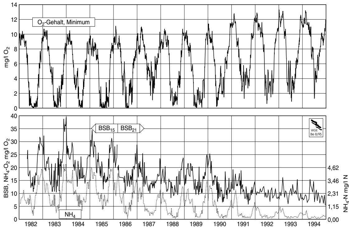
Abb. 10: Tageminima der Sauerstoffgehalte aus kontinuierlichen Messungen, BSB 15 /BSB 21 - und Ammoniumgehalte aus wöchentlichen Einzelproben (ab 1992 14-täglich) - Elbe bei Seemannshöft (Strom-km 628,8)
