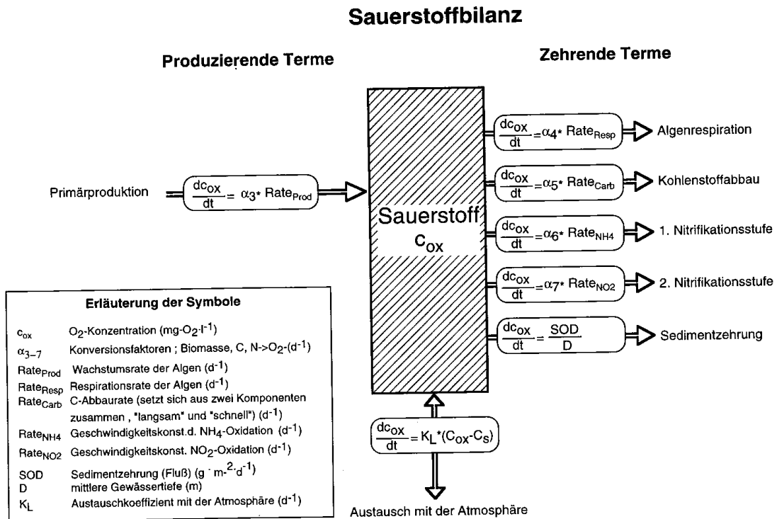
Abb. 25a: Im Modell berücksichtigte Prozesse des Teilsystems „Sauerstoff“
