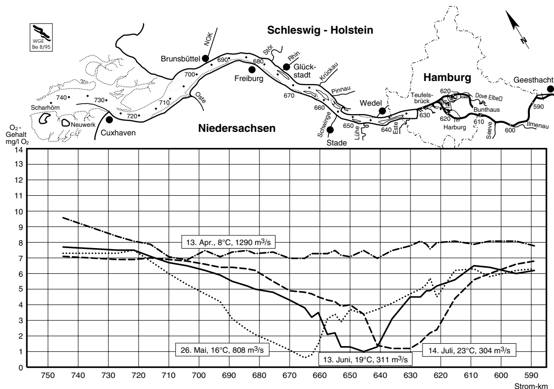
Abb. 8: Sauerstoff-Längsprofile der Tideelbe - Frühjahrsentwicklung 1983
