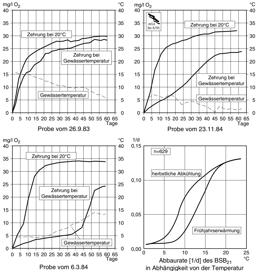
Abb. 5: Sauerstoffzehrung bei Gewässertemperatur und 20°C und errechnete Abbauraten des BSB 21 , Elbwasserproben bei Seemannshöft (Strom-km 628,8), April 1983 bis März 1985.
