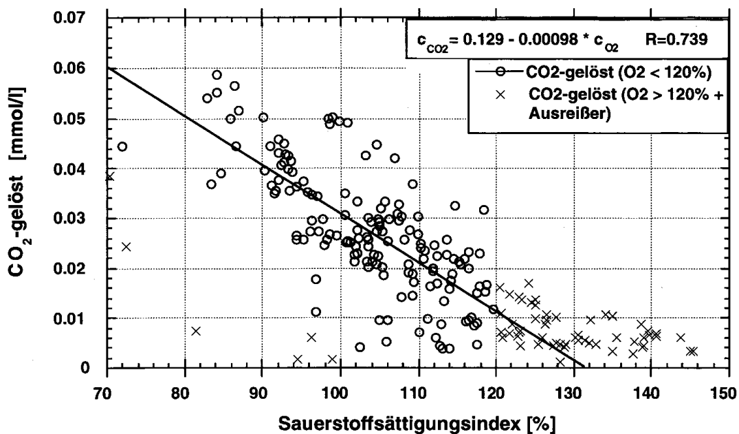
Abb. 13: Korrelation zwischen O 2 -Sättigungsindex und gelöstem CO 2 von März bis Oktober 1995 (Für die Korrelationsgerade wurden nur Werte herangezogen, bei denen der Sauerstoffsättigungsindex unter 120 % lag)
