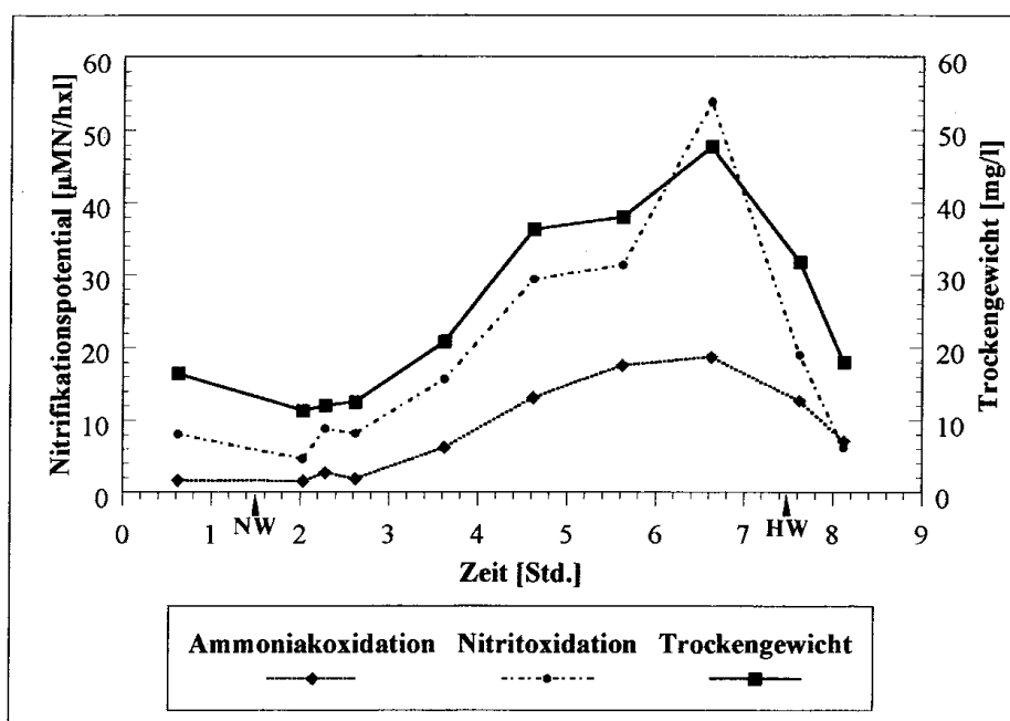
Abb. 6: Tideabhängiger Verlauf des Ammoniak- und Nitritoxidationspotentials sowie des Trockengewichtes von Wasserproben der Station Nienstedten am 7. November 1988. HW = Tide-Hochwasser, NW = Tide-Niedrigwasser. Aus: Sowitzki (1992)
