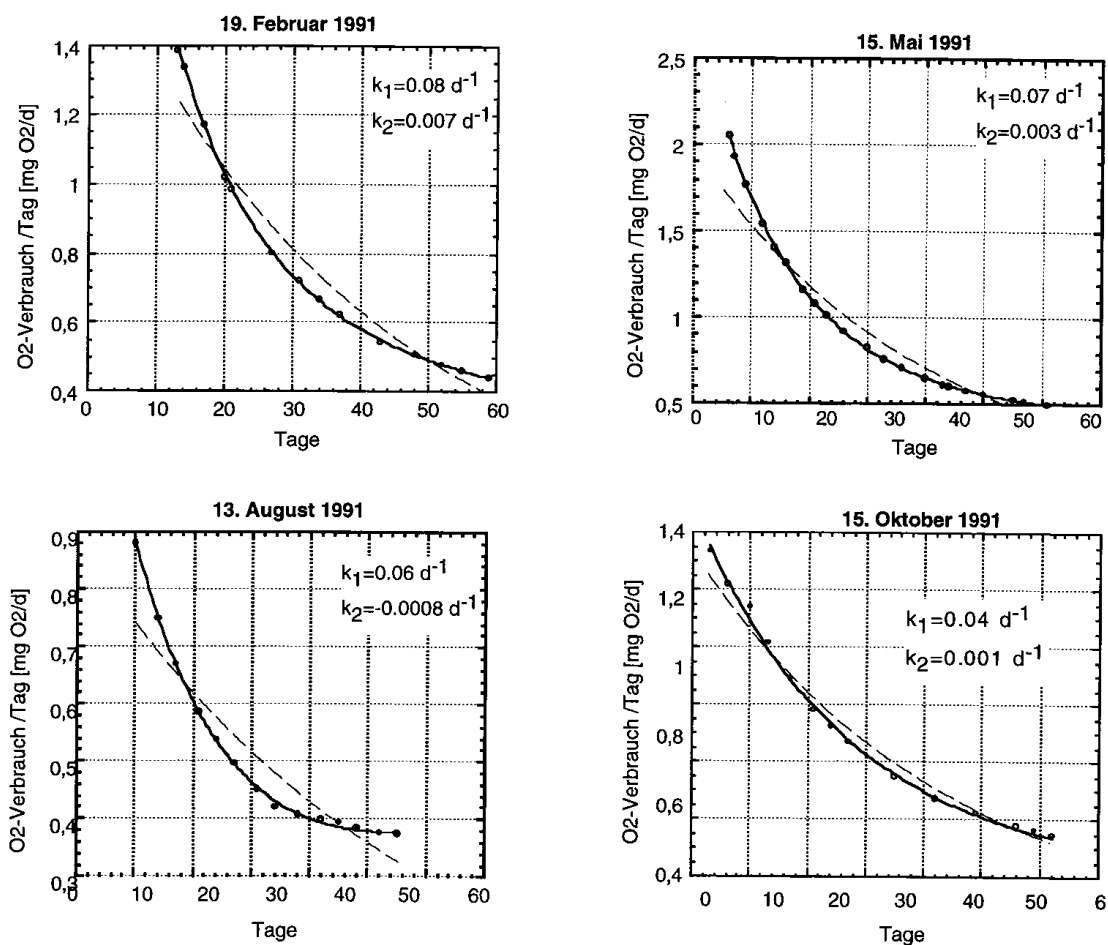
Abb. 26: BSB-Werte (auf ein Zeitintervall von 24 Stunden normiert) – Elbe bei Elbstorf (Inkubationen im Dunkeln bei 20 °C), Februar bis September 1991 –. Die Kurvenanpassungen (Linien) erfolgten über eine bzw. zwei e-Funktionen. (Messungen ARGE Elbe, M. BERGEMANN, persönl. Mittlg.)
