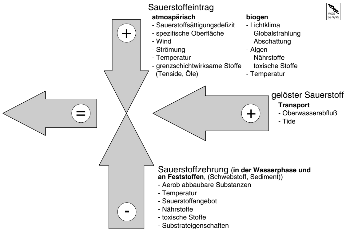
Abb. 2: Die Einflußgrößen auf den Sauerstoffgehalt eines Fließgewässers
