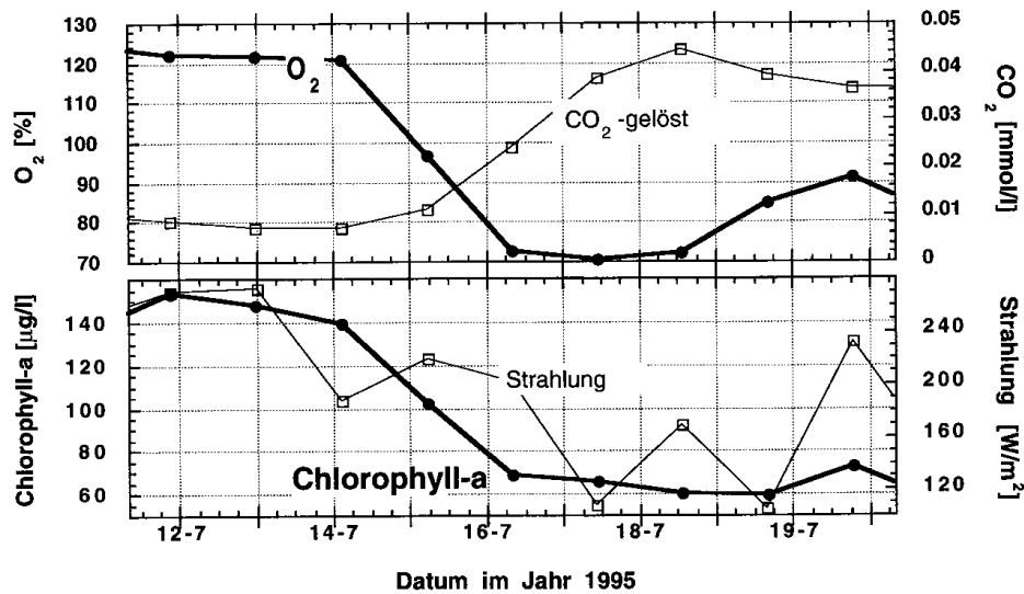
Abb. 14: Typisches Beispiel eines O 2 -Einbruchs Mitte Juli 1995 (Tagesmittelwerte bzw. Tagesmaxima für Chlorophyll-a)
