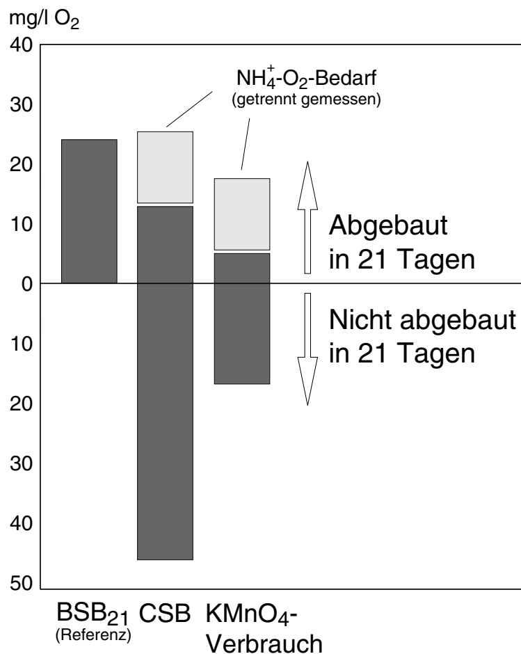
Abb. 4: CSB und \text{KMnO}_4 -Verbrauch (PV) sofort und nach 21 Tagen Inkubationszeit, \text{BSB}_{21} und Ammonium-Sauerstoffäquivalent - Elbwasserprobe oberhalb von Elbstorf (Strom-km 589, 16.8.84)
