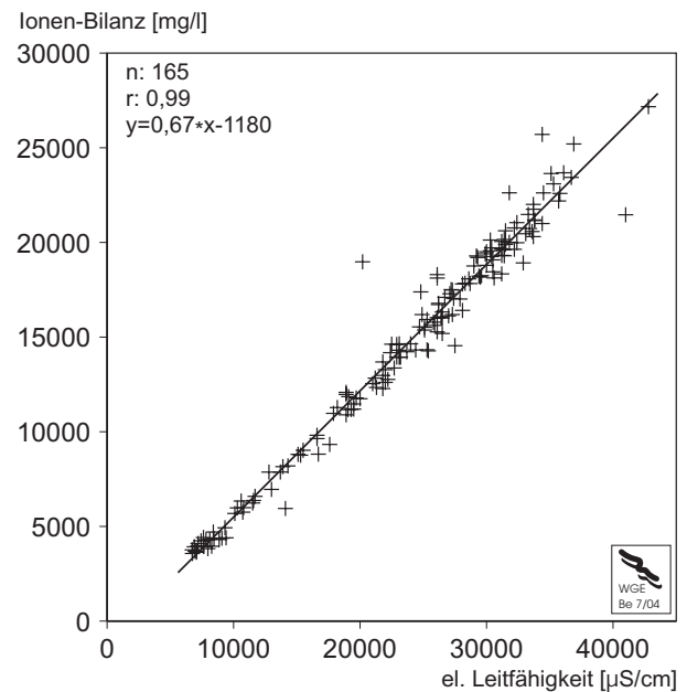
Abb. 4 Verhältnis der elektrischen Leitfähigkeit (25°C) zu der Ionen-Bilanz im Brackwasserbereich der Elbe (Brunsbüttel-Cuxhaven) - 1994-2003
