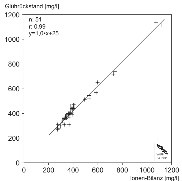
Abb. 2 Verhältnis der Ionen-Bilanz zu dem Glührückstand der Elbe im Süßwasserbereich (Schmilka-Hamburg) - 1964-1990
