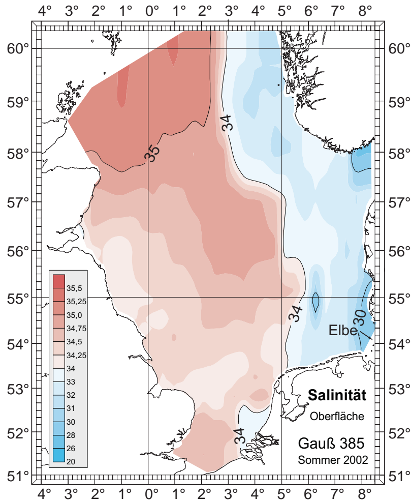
Abb. 1 Salzgehalt der Nordsee, Messungen des Messschiffes „Gauß“ im Sommer 2002 (Quelle Bundesamt für Seeschifffahrt und Hydrographie)
