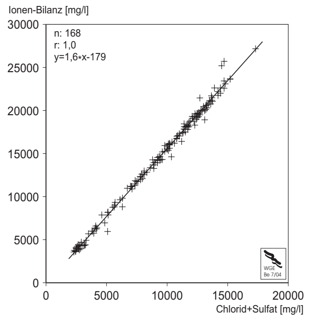
Abb. 8 Verhältnis der Chlorid+Sulfat-Gehalte zu der Ionen-Bilanz der Elbe im Brackwasserbereich (Brunsbüttel-Cuxhaven) - 1994-2003
