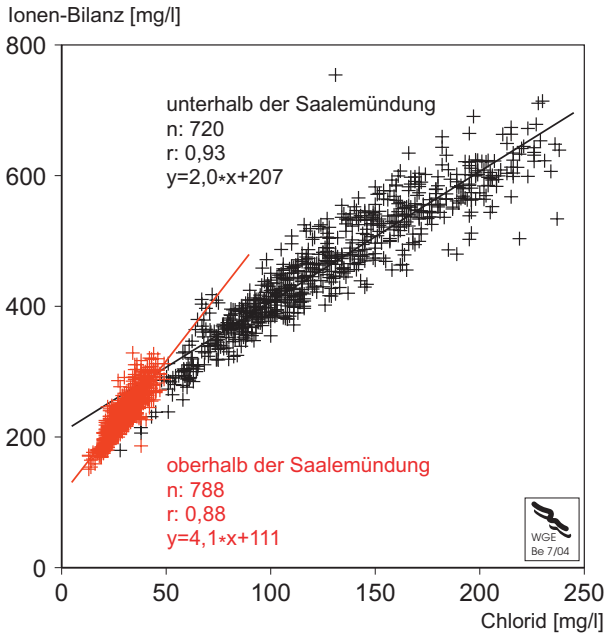
Abb. 5 Verhältnis der Chlorid-Gehalte zu der Ionen-Bilanz der Elbe im Süßwasserbereich (Schmilka-Hamburg) - 1994-2003
