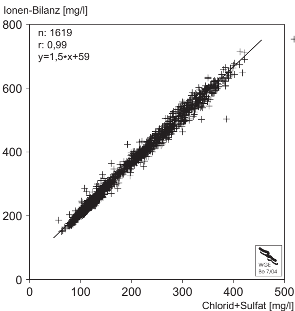
Abb. 7 Verhältnis der Chlorid+Sulfat-Gehalte zu der Ionen-Bilanz der Elbe im Süßwasserbereich (Schmilka-Hamburg) - 1994-2003
