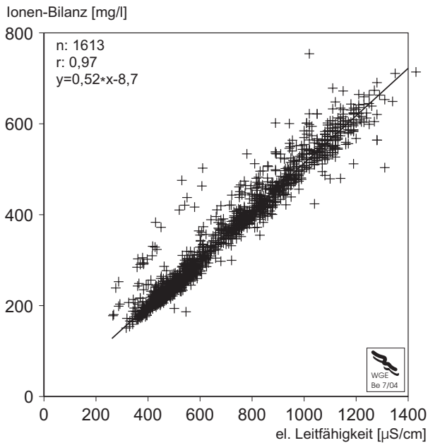
Abb. 3 Verhältnis der elektrischen Leitfähigkeit (25°C) zu der Ionen-Bilanz im Süßwasserbereich der Elbe (Schmilka-Hamburg) - 1994-2003
