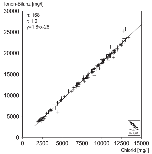
Abb. 6 Verhältnis der Chlorid-Gehalte zu der Ionen-Bilanz der Elbe im Brackwasserbereich (Brunsbüttel-Cuxhaven) - 1994-2003
