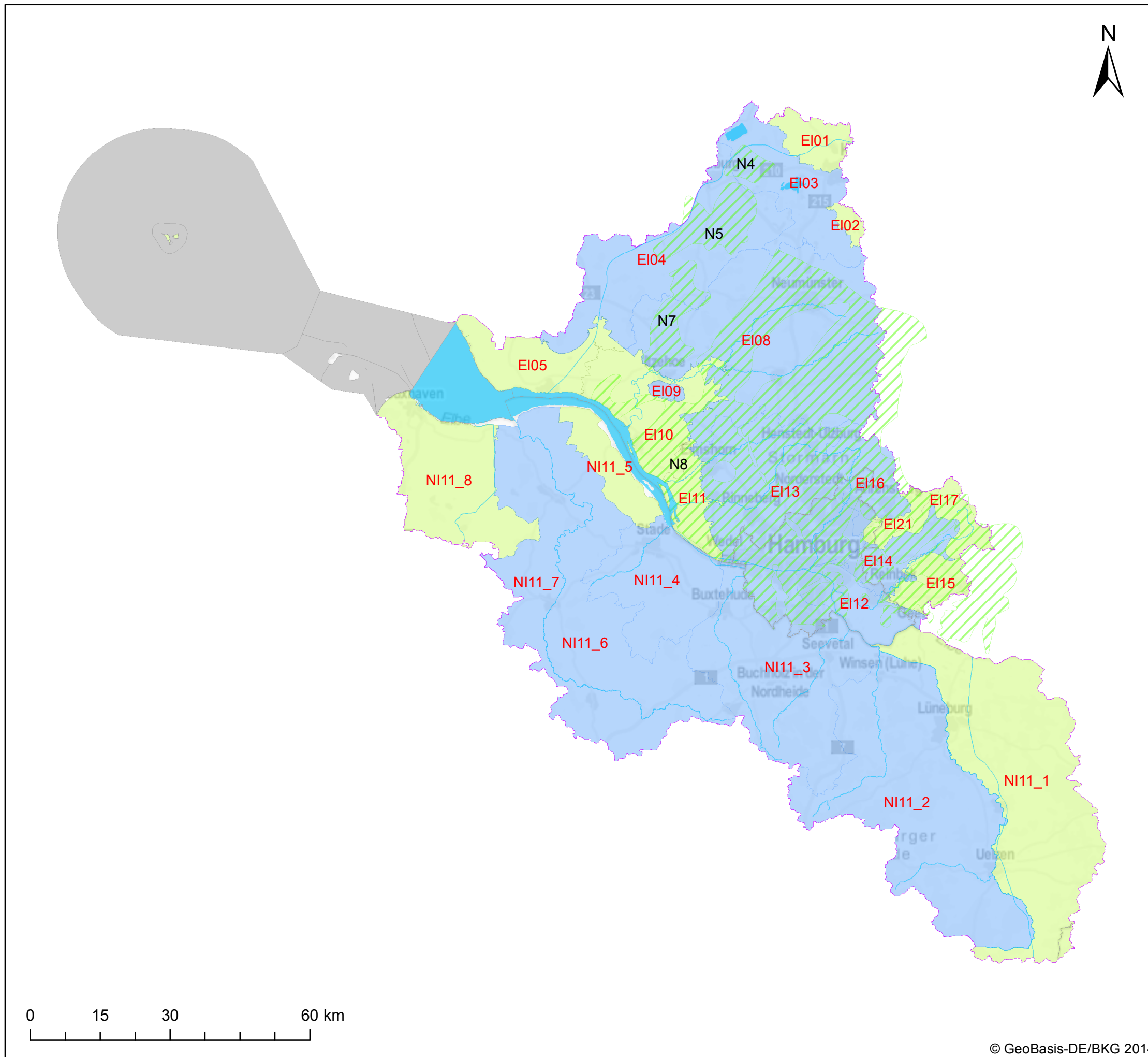
KOR Tideelbe - Karte 5.4: Umweltziele der Grundwasserkörper - Chemie
