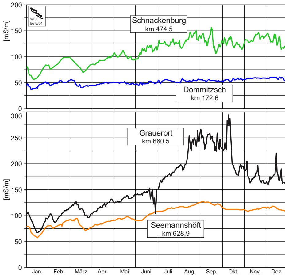
Abb. 3 Elektrische Leitfähigkeit bei 25°C (Tagesmittelwerte) der Elbe 2003
