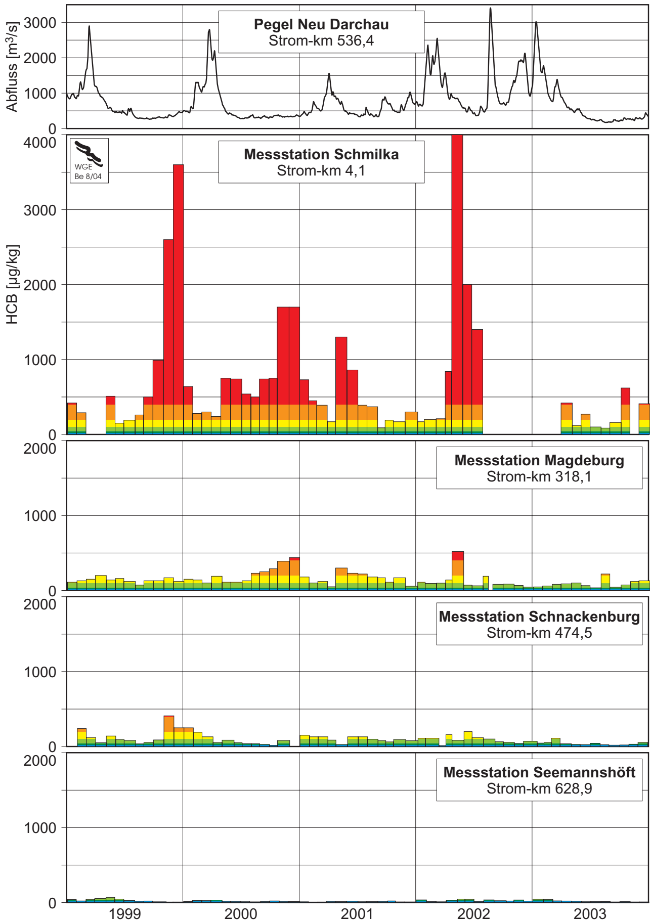
Abb. 20 Hexachlorbenzen in frischen schwebstoffbürtigen Sedimenten - 1999-2003
