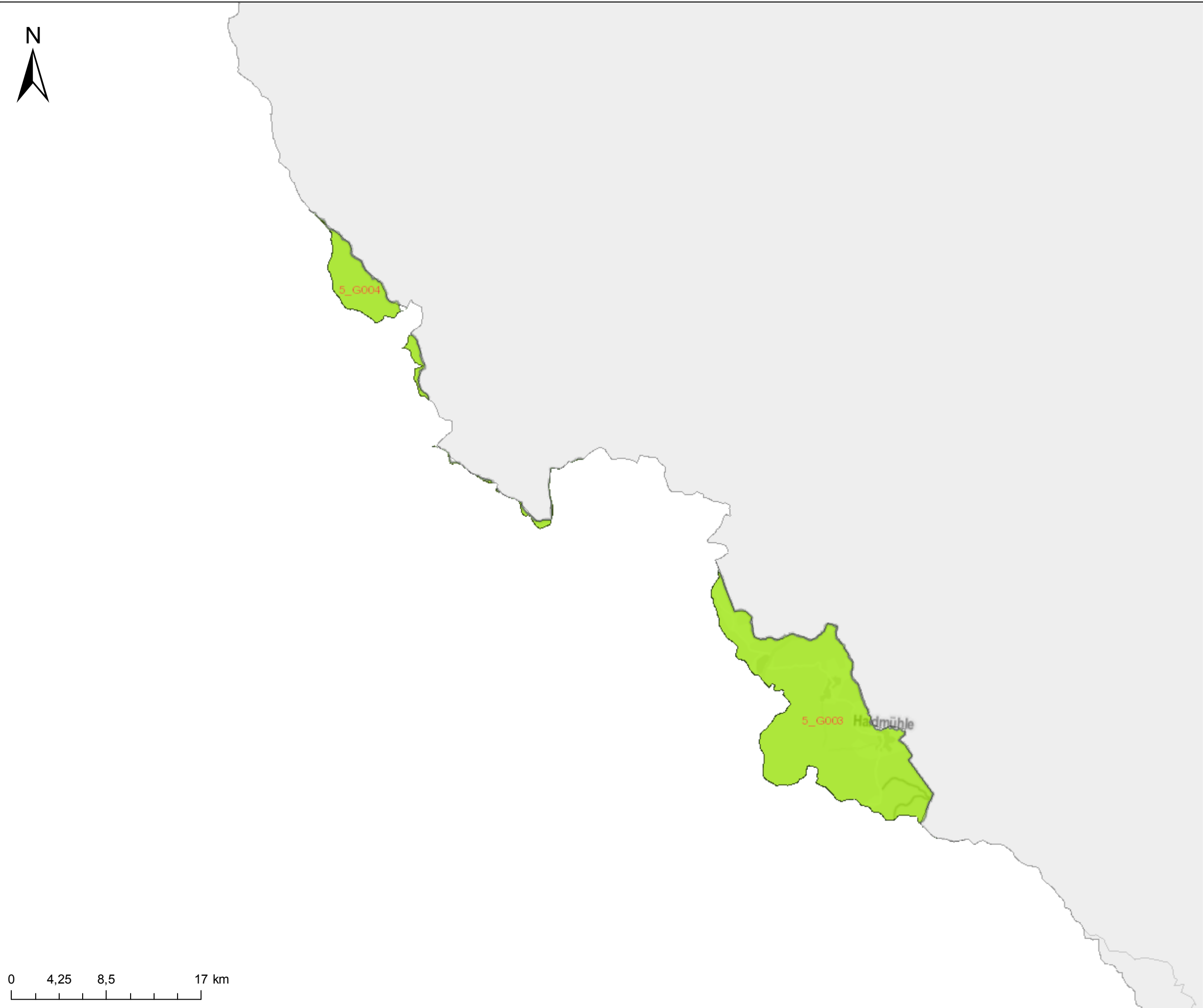
KOR Obere Moldau - Karte 4.6.2: Chemischer Zustand der Grundwasserkörper hinsichtlich Pestiziden
