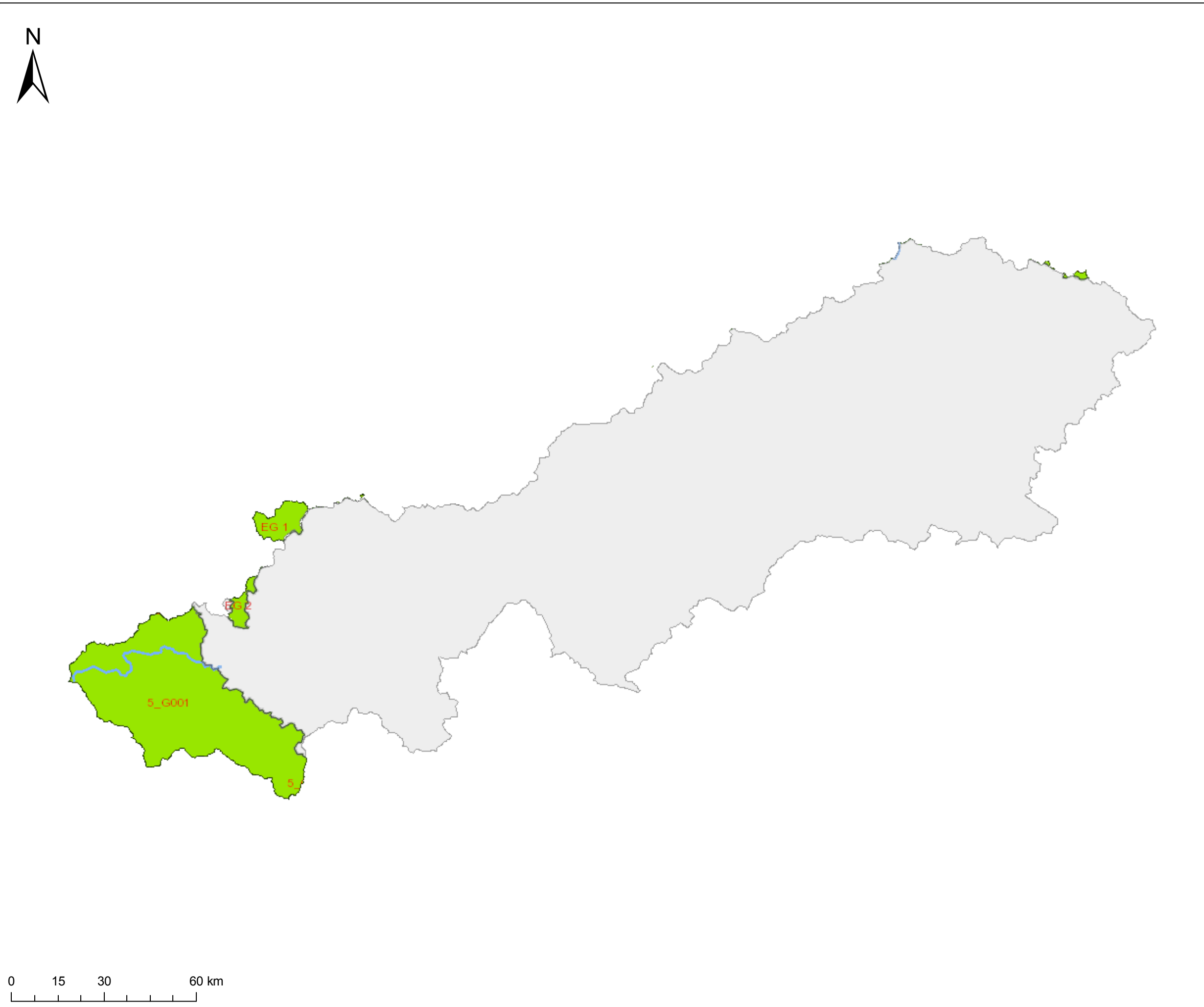
KOR Eger und Untere Elbe - Karte 4.6.2: Chemischer Zustand der Grundwasserkörper hinsichtlich Pestiziden
